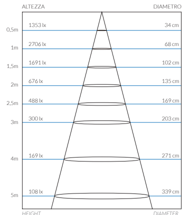
CONO DI LUCE 36° 36° CONE OF LIGHT
