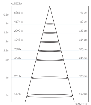
CONO DI LUCE 36° 36° CONE OF LIGHT
