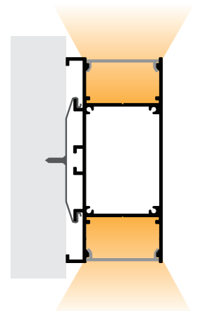
Installazione a parete wall / ceiling fixing
